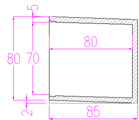
SEZIONE
