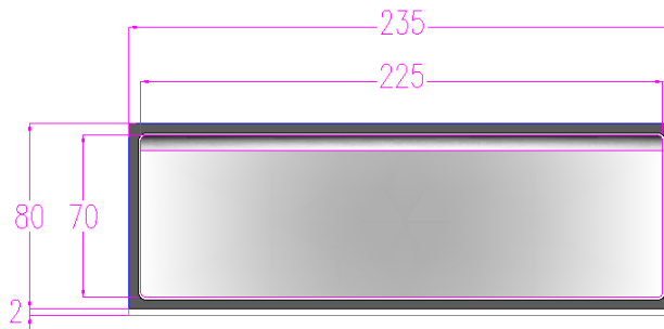
FRONTALE
