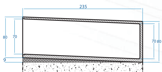
Sezione Longitudinale
