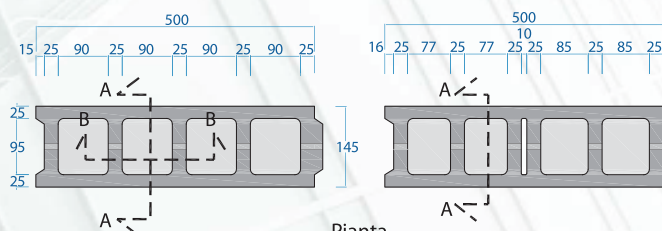
Pianta
