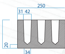
Sezione
