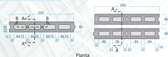
Pianta
