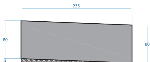
Vista Laterale
