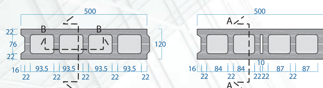
Pianta
