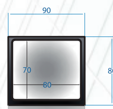
Vista Frontale
