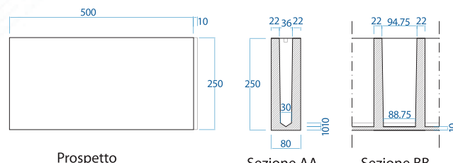
Prospetto
