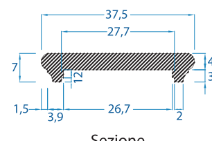
Sezione
