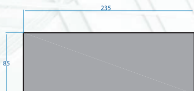
Vista Superiore
